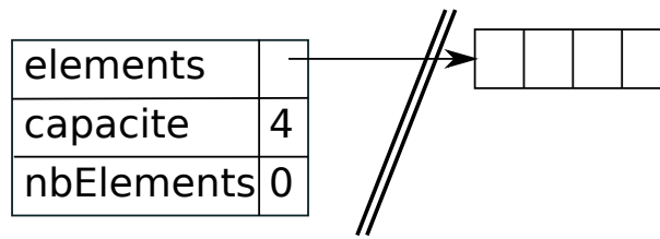
FIGURE 10 – Exemple de représentation de la classe Tableau
