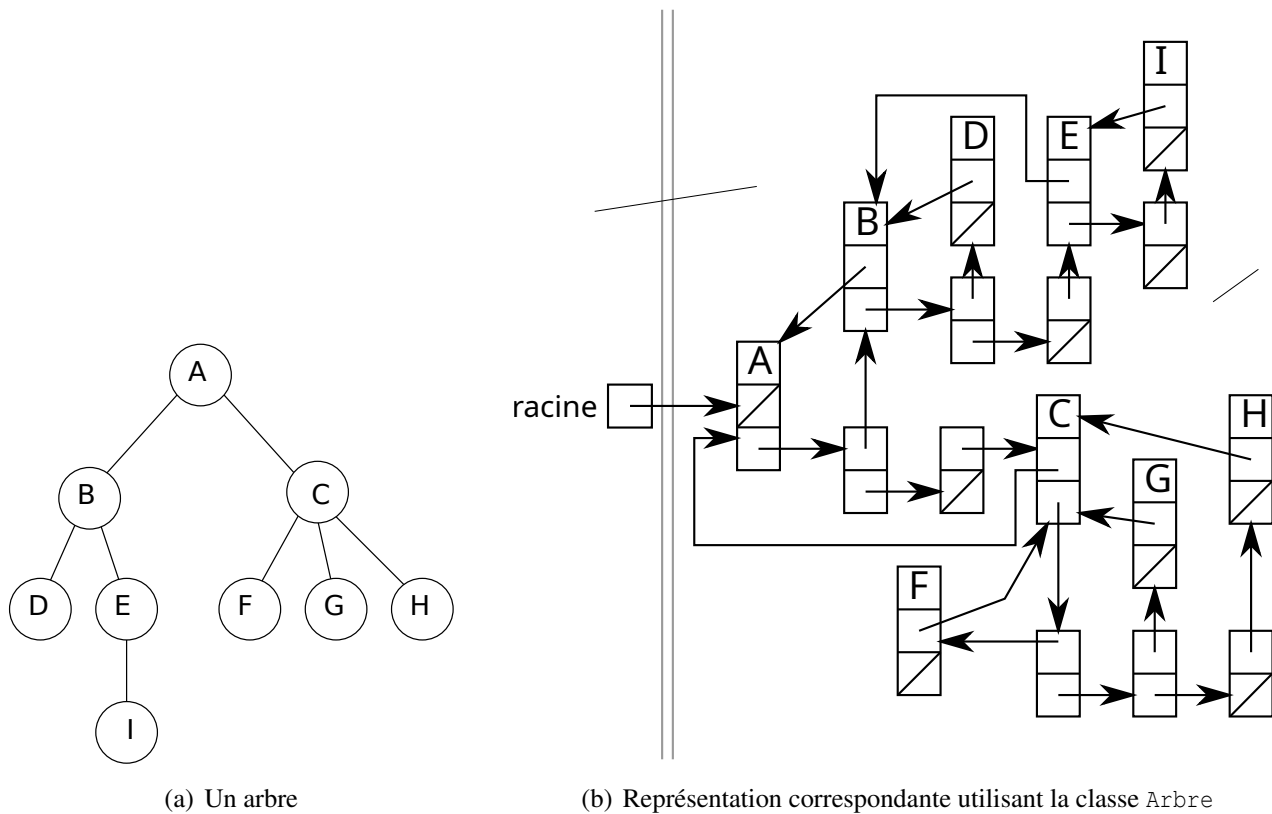
FIGURE 25 – Exemple de représentation
