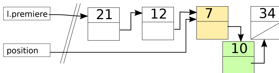
FIGURE 18 – Insertion après une cellule
