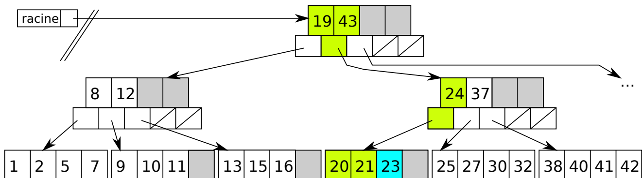
FIGURE 43 – Exemple de recherche de l'élément 23 dans un arbre B
