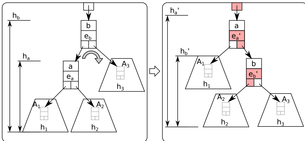
FIGURE 37 – Rotation gauche-droite
