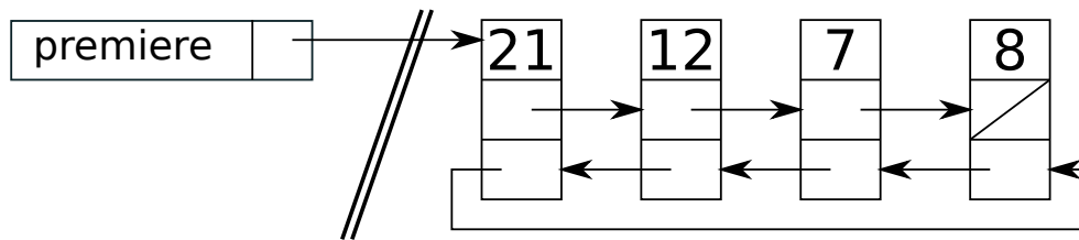
FIGURE 22 – Liste doublement chaînée
