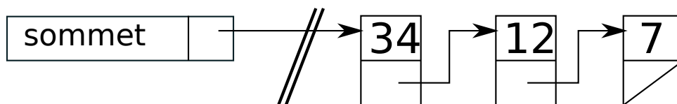
FIGURE 12 – Représentation d'une pile à l'aide de cellules chaînées
