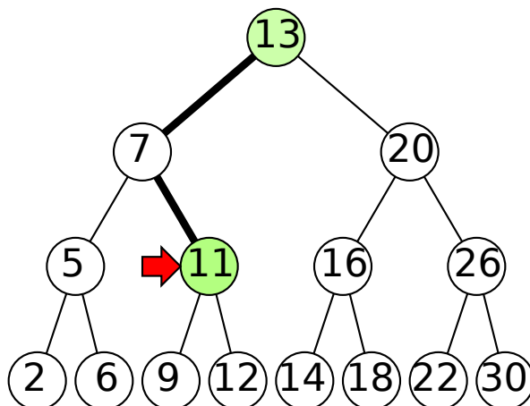
FIGURE 38 – État d'itération d'un parcours en inordre
