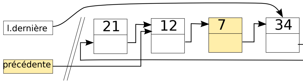
FIGURE 21 – Liste chaînée avec un concept de pointeurs décalés (sur le précédent)
